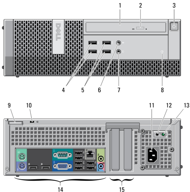
Rysunek 3. Panel przedni i tylny: obudowa typu SFF
